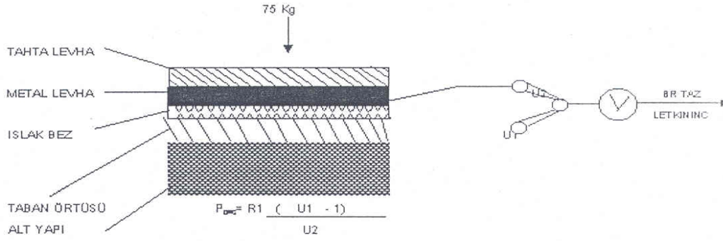
Şekil 20 – Zemin yalıtıkanlık direncinin ölçülmesi
